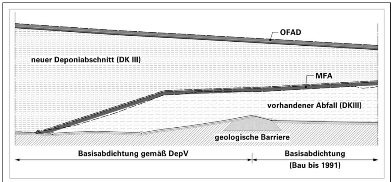
Abbildung 5: Querschnittsdarstellung zur Variante 2 - „horizontale Basisanbindung“
