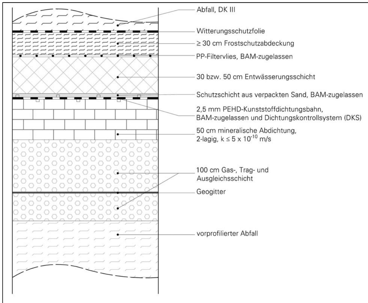
Abbildung 7: Aufbau der Multifunktionalen Abdichtung der Deponie Ihlenberg
