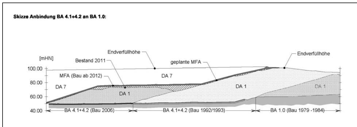
Abbildung 3: Schnittdarstellung „Trennung DA 1 / DA 7 – Anbindung der BA 4.1+4.2 an BA 1.0“
