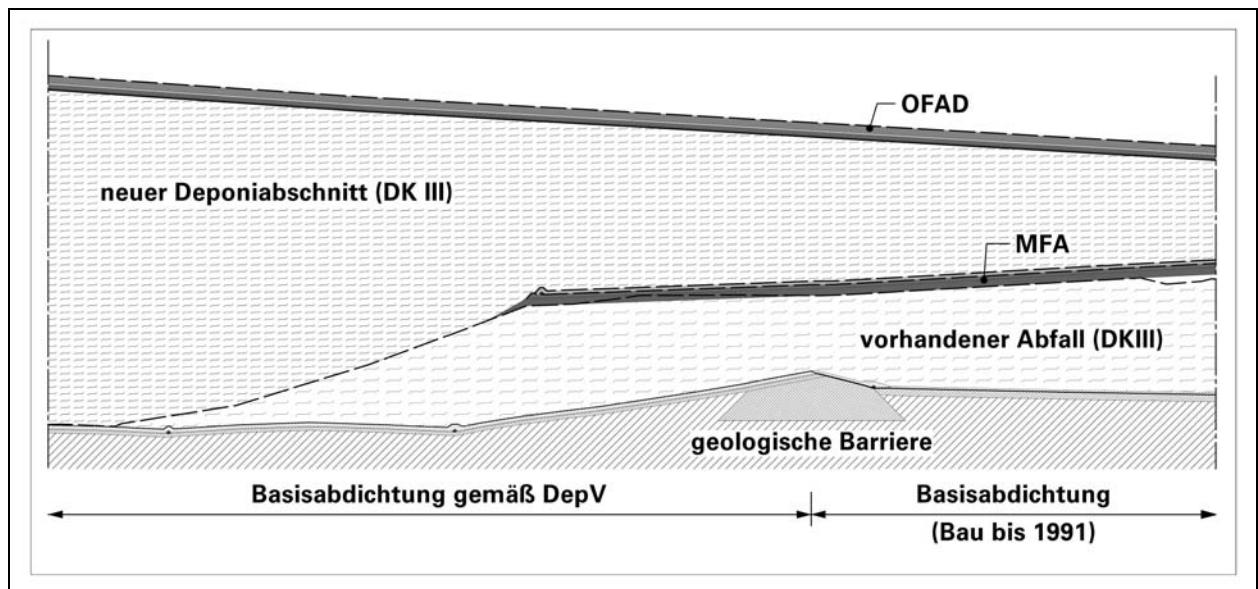
Abbildung 4: Querschnittsdarstellung zur Variante 1 - „Schirmlösung“
