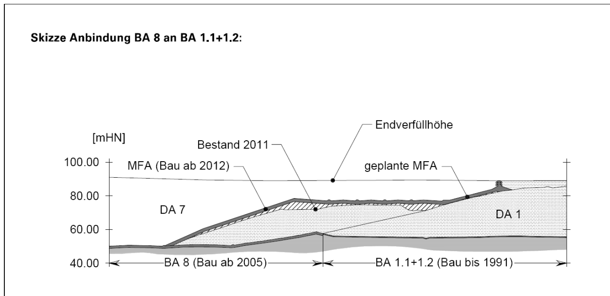
Abbildung 2: Schnittdarstellung „Trennung DA 1 / DA 7- Anbindung des BA 8 an BA 1.1+1.2“
