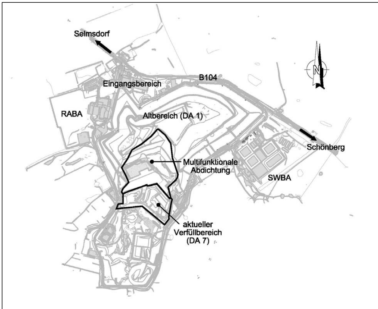
Abbildung 1: Übersichtslageplan „Standort Ihlenberg – Lage der MFA“
