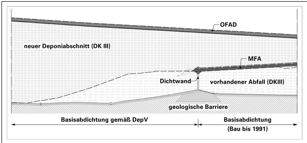
Abbildung 6: Querschnittsdarstellung zur Variante 3 - „vertikale Basisanbindung“
