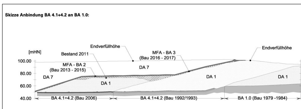
Abbildung 1 Deponie Ihlenberg, Schnittdarstellung Trennung DA 1 / DA 7
