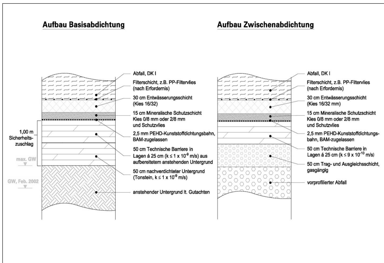
Abbildung 5 Deponie Reesberg, Abdichtungssysteme der DaD gemäß Planfeststellungsantrag (Neudeponieabschnitt der DK I)
