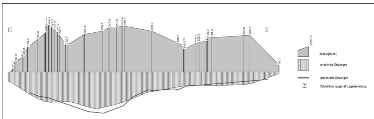
Abbildung 3 Deponie Ihlenberg, Graphische Darstellung zur Auswertung von Setzungsmessungen und Setzungsprognosen an SM 5
