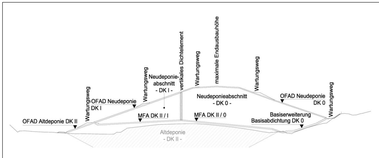
Abbildung 6 Deponie Fludersbach, Schnittdarstellung
