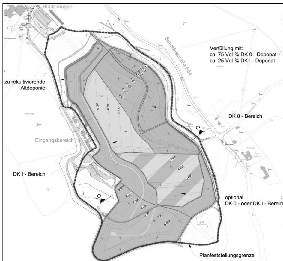
Abbildung 8 Deponie Fludersbach, Lageplan mit Kennzeichnung der Deponieabschnitte
