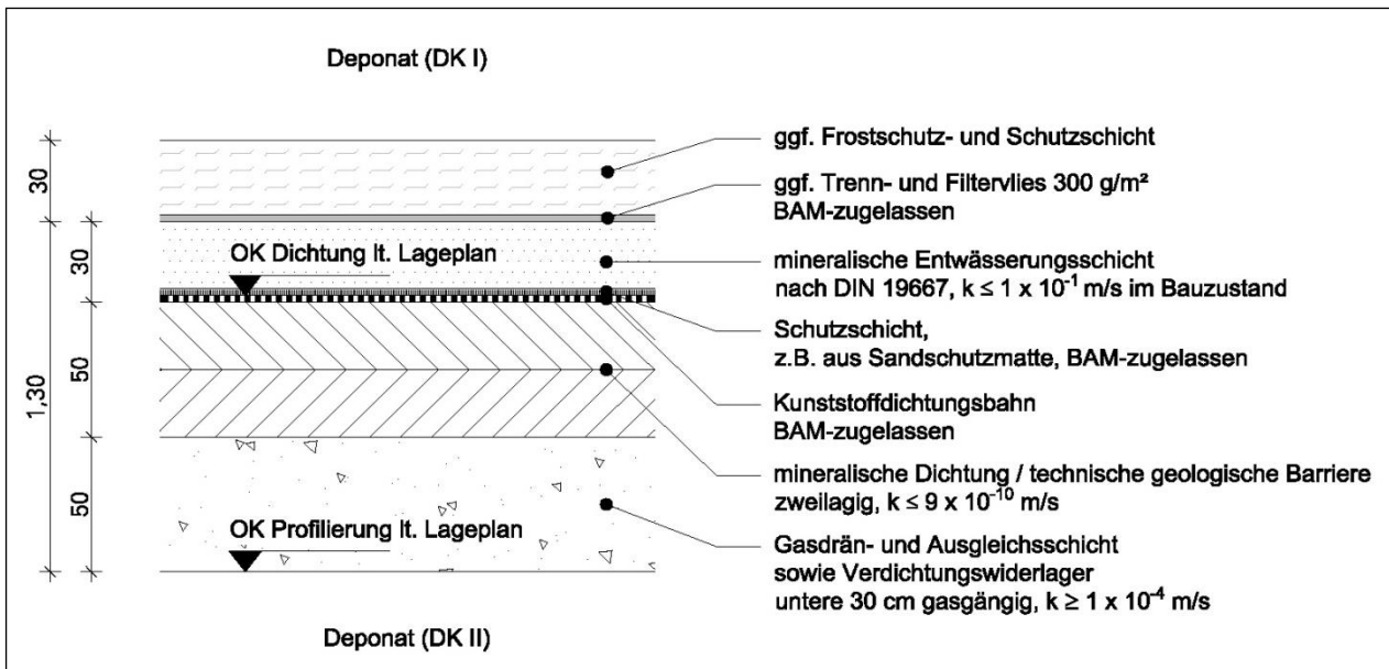
Abbildung 7 Deponie Fludersbach, Abdichtungssystem der MFA (Neudeponieabschnitt der DK I)
