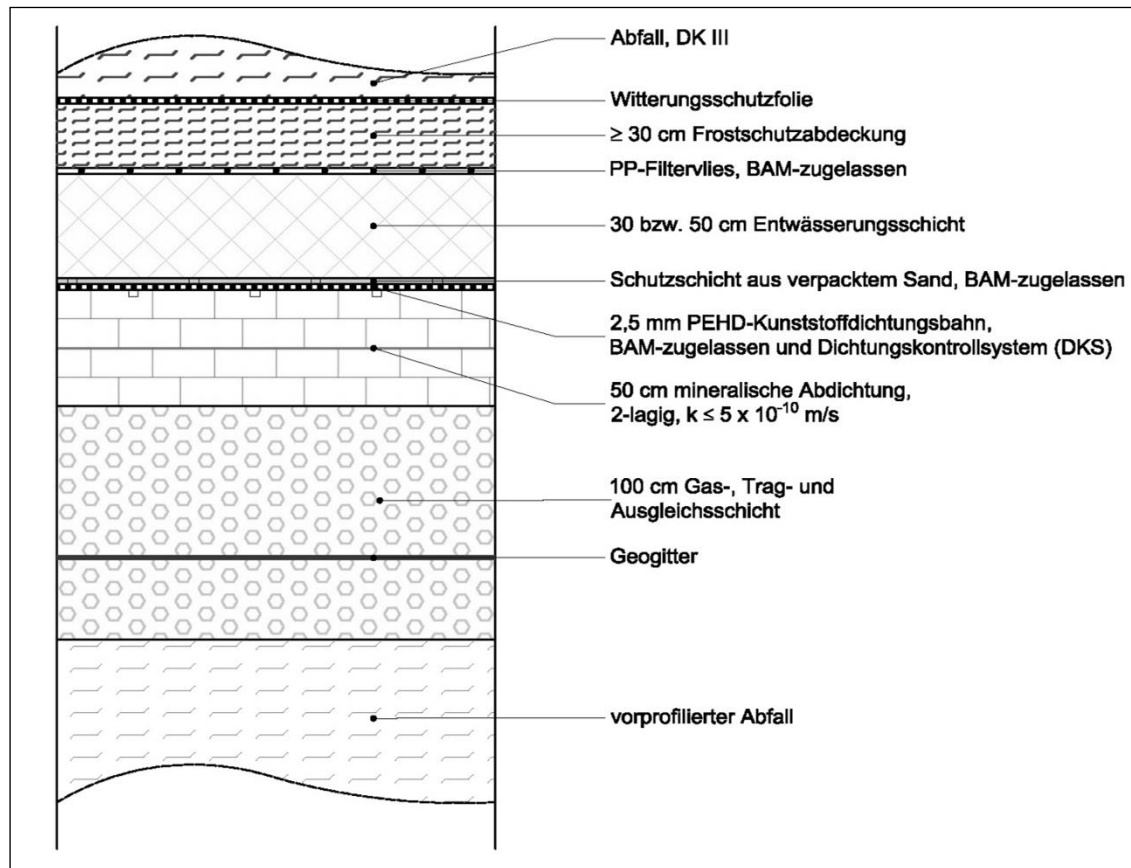
Abbildung 2 Deponie Ihlenberg, Abdichtungssystem der MFA (DK III)
