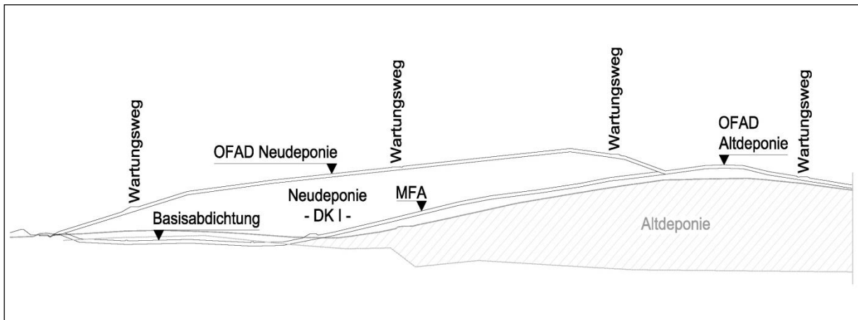
Abbildung 4 Deponie Reesberg, Querschnitt im Anlehnungsbereich
